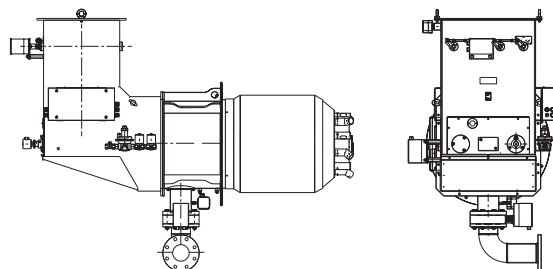
DB 16-20 (версия A180-воздухозабор сверху)
