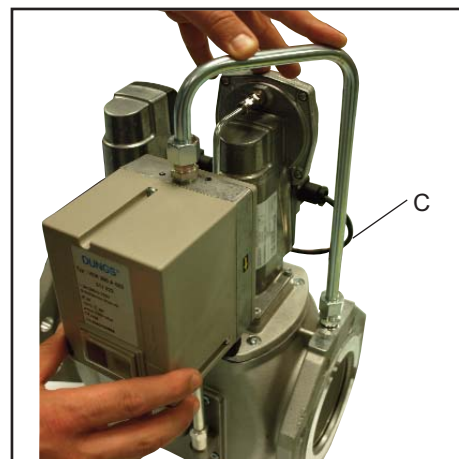
6- Install the pipe. - Montare il tubo. - Monter le tube. - Montar el tubo. - Установить трубу.
