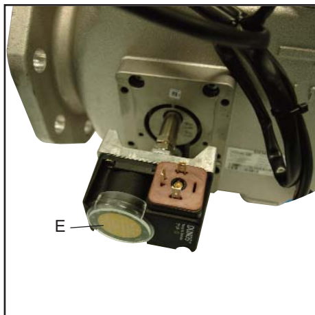
5- Install the gas pressure switch. - Montare il pressostato gas. - Monter le pressostat gaz. - Montar el presóstat de gas. - Установить Функция реле давления газа.
