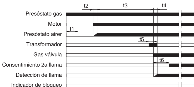
Ciclo de funcionamiento normal
