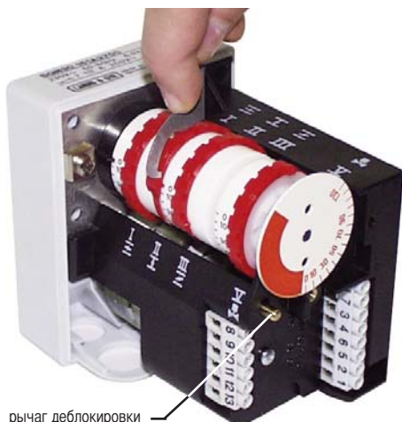
рычаг деблокировки
