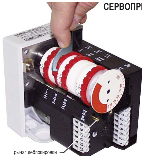
рычаг деблокировки
