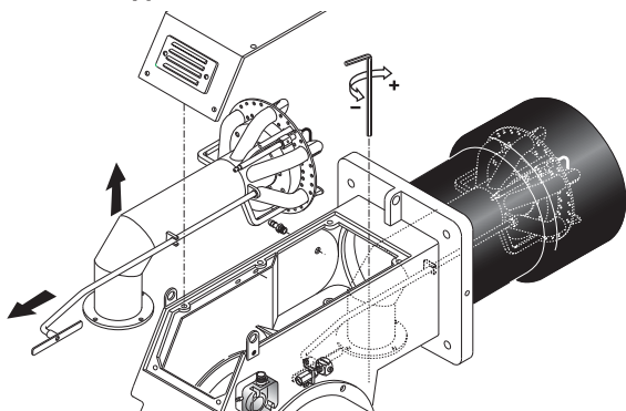
ДЕМОНТАЖ ОГНЕВОЙ ГОЛОВКИ
