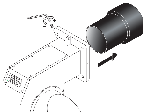
ДЕМОНТАЖ СТАКАНА
