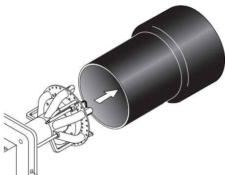
DEMONTAGE DE GUEULARD
