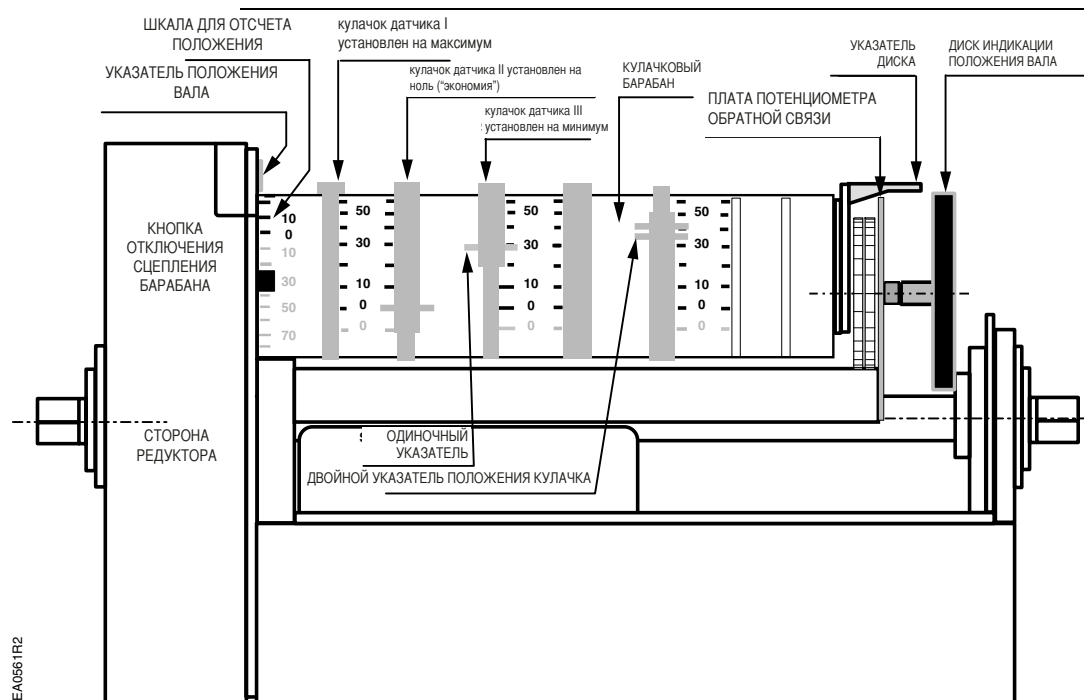
Рис. 6. Расположение компонентов кулачкового барабана привода SQM5...
