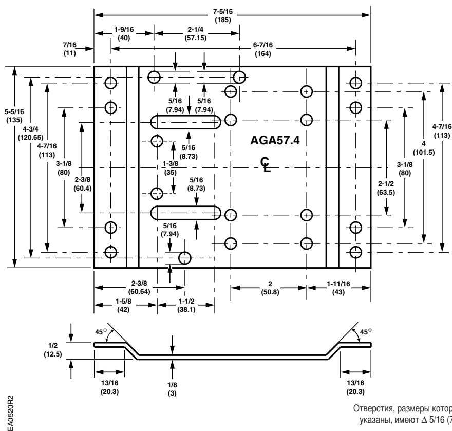
Рис. 30. Монтажная скоба AGA57.4
