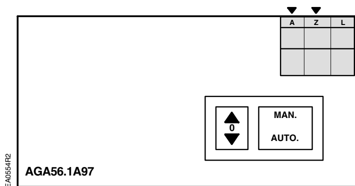
Рис. 8. Плата AGA56.1A97
